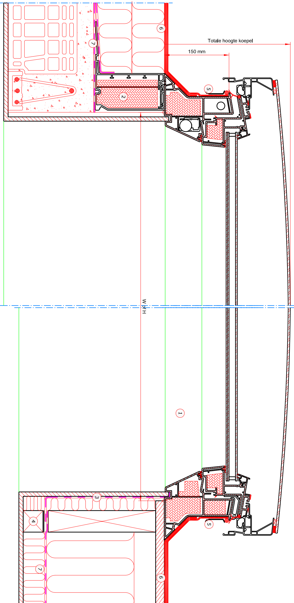
Doorsnede A-A 1:5
